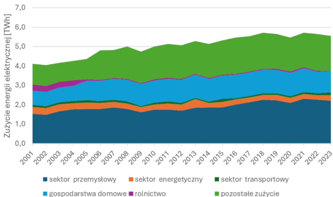
Ryc. 49 Zużycie energii elektrycznej w województwie podkarpackim w latach 2001–2023
